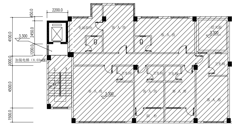
2层平面图
