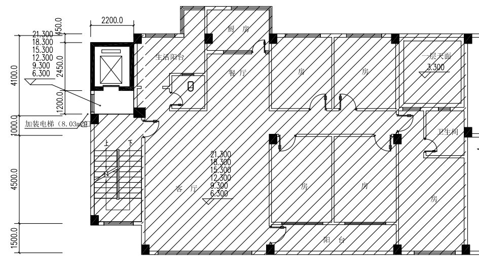
3-8层平面图
