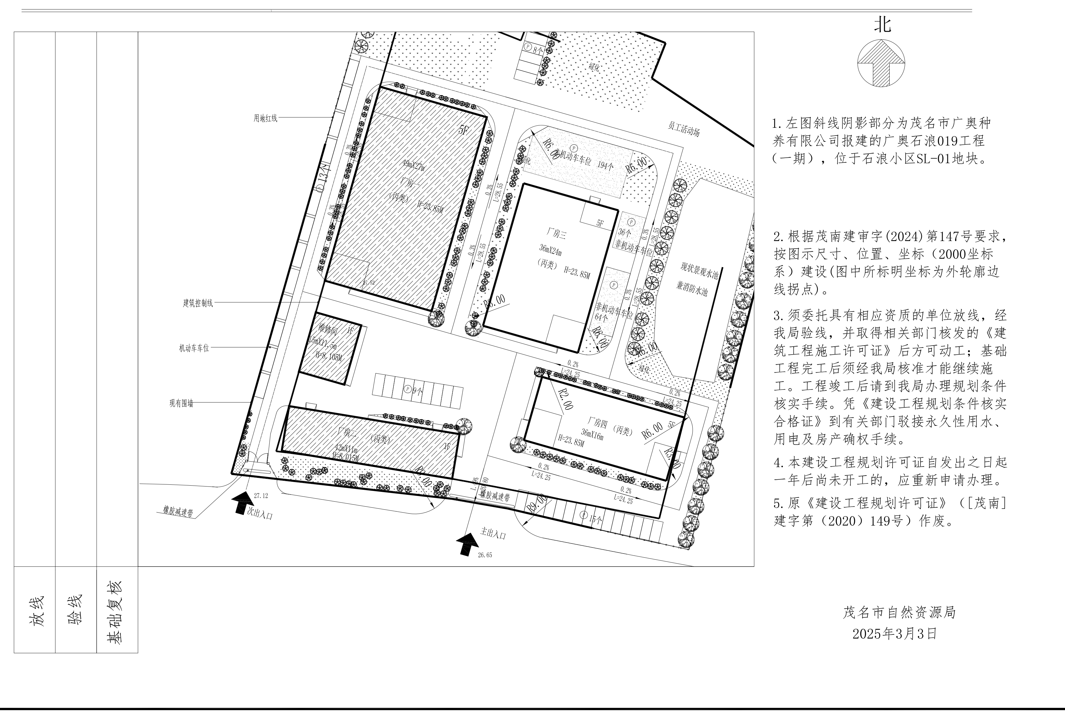
建设工程放线平面图
