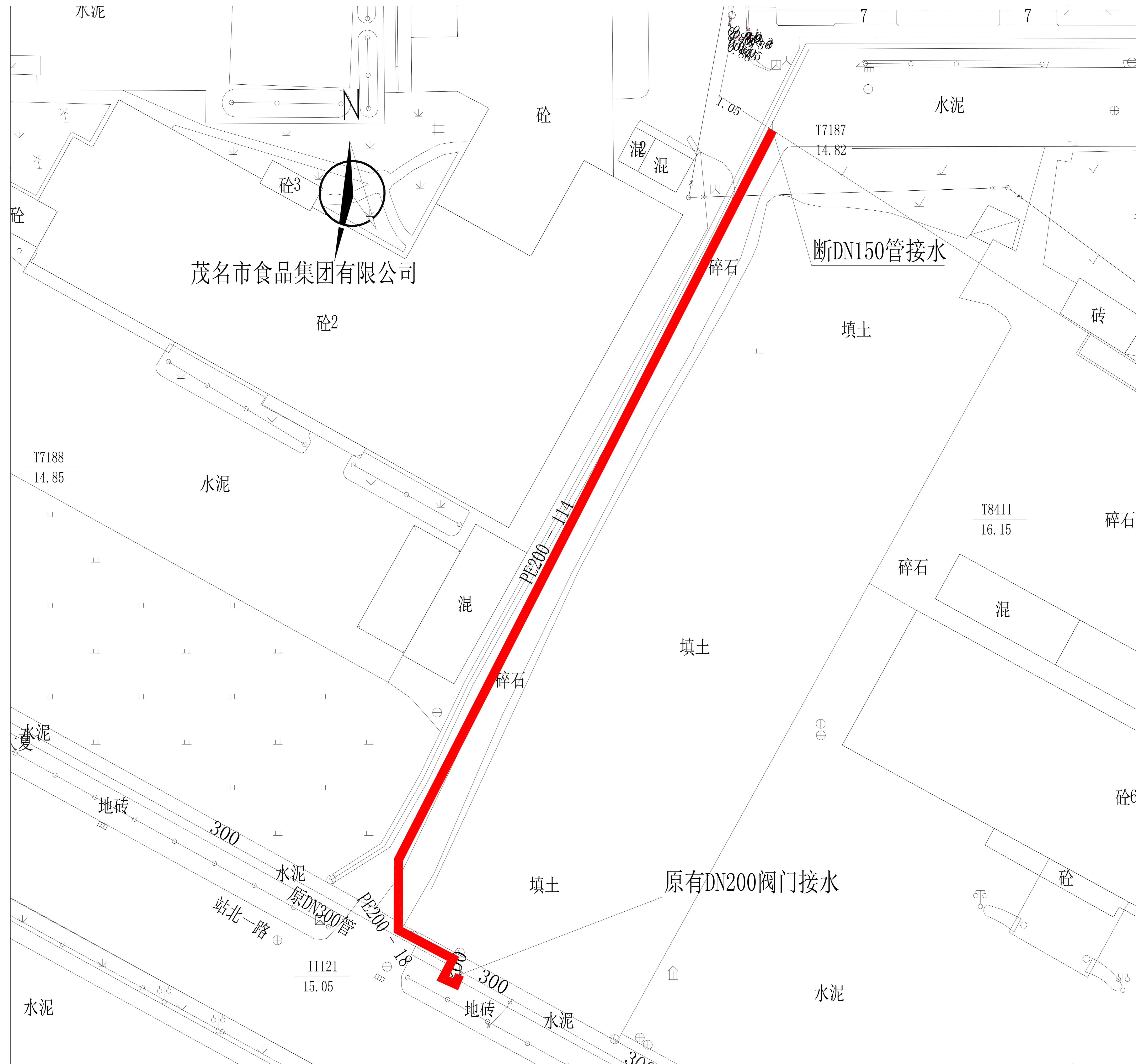
总平面图
