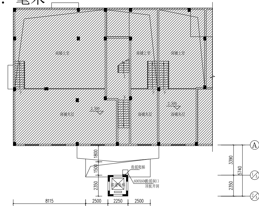
夹层平面图
