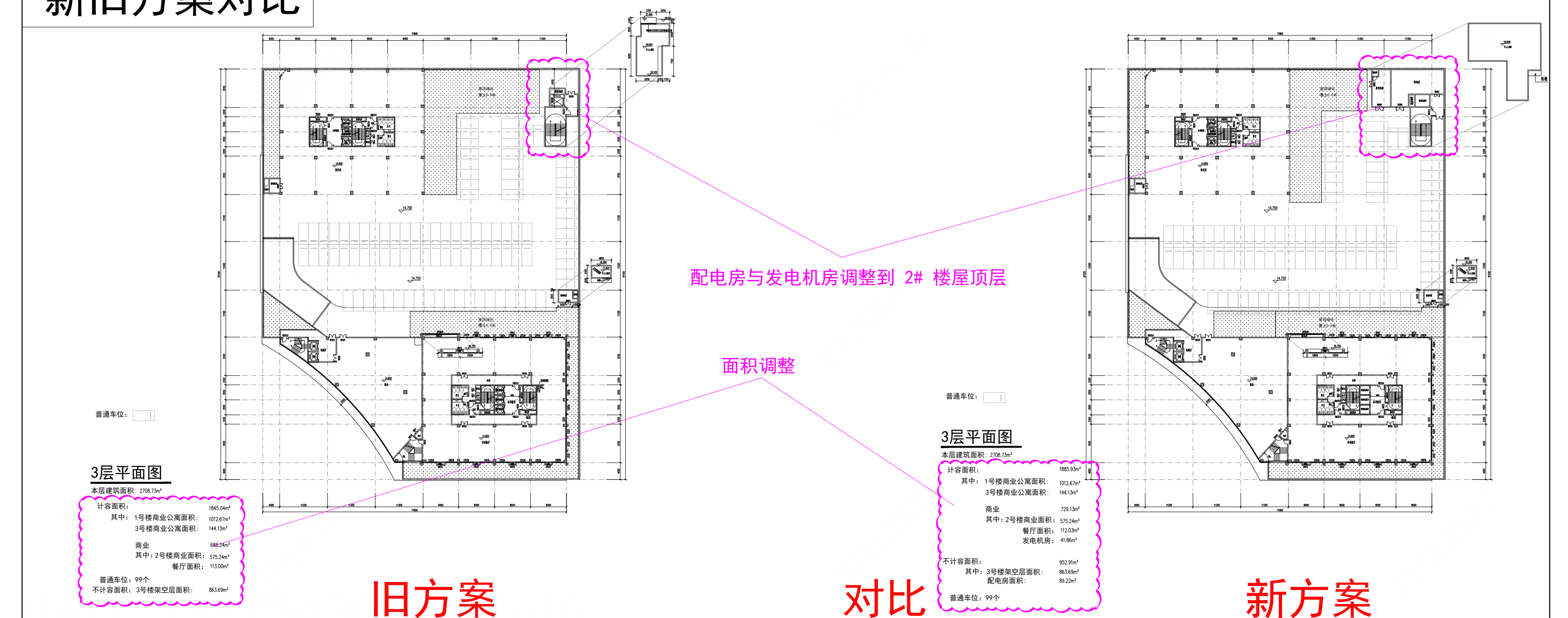
修改新旧对比三层平面图
