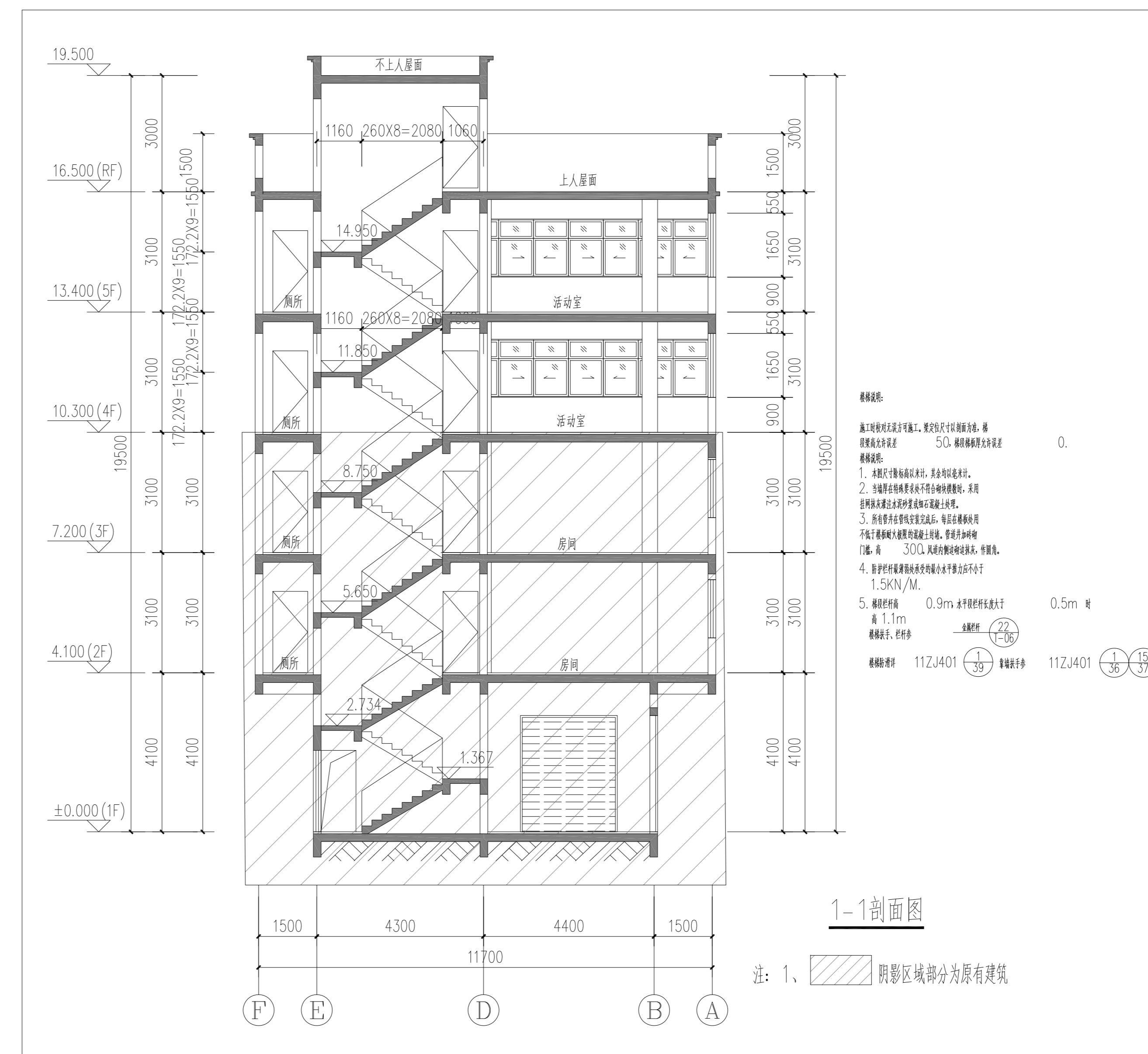
剖面图
