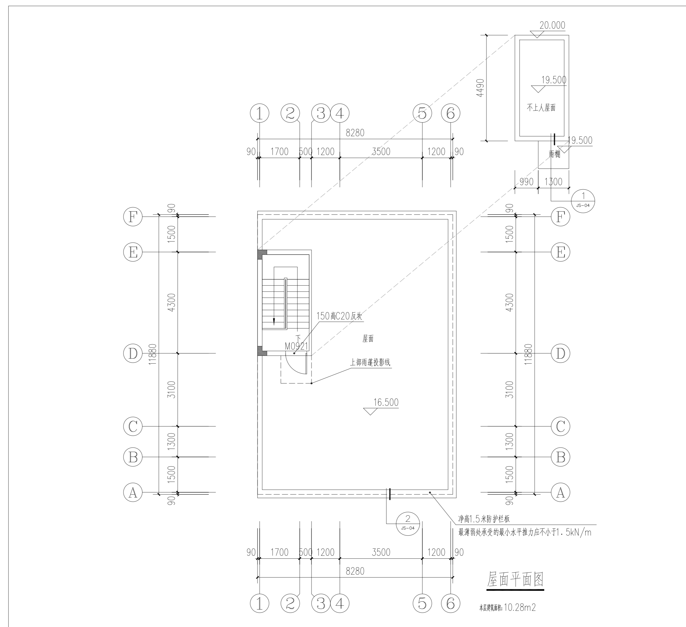
屋面平面图
