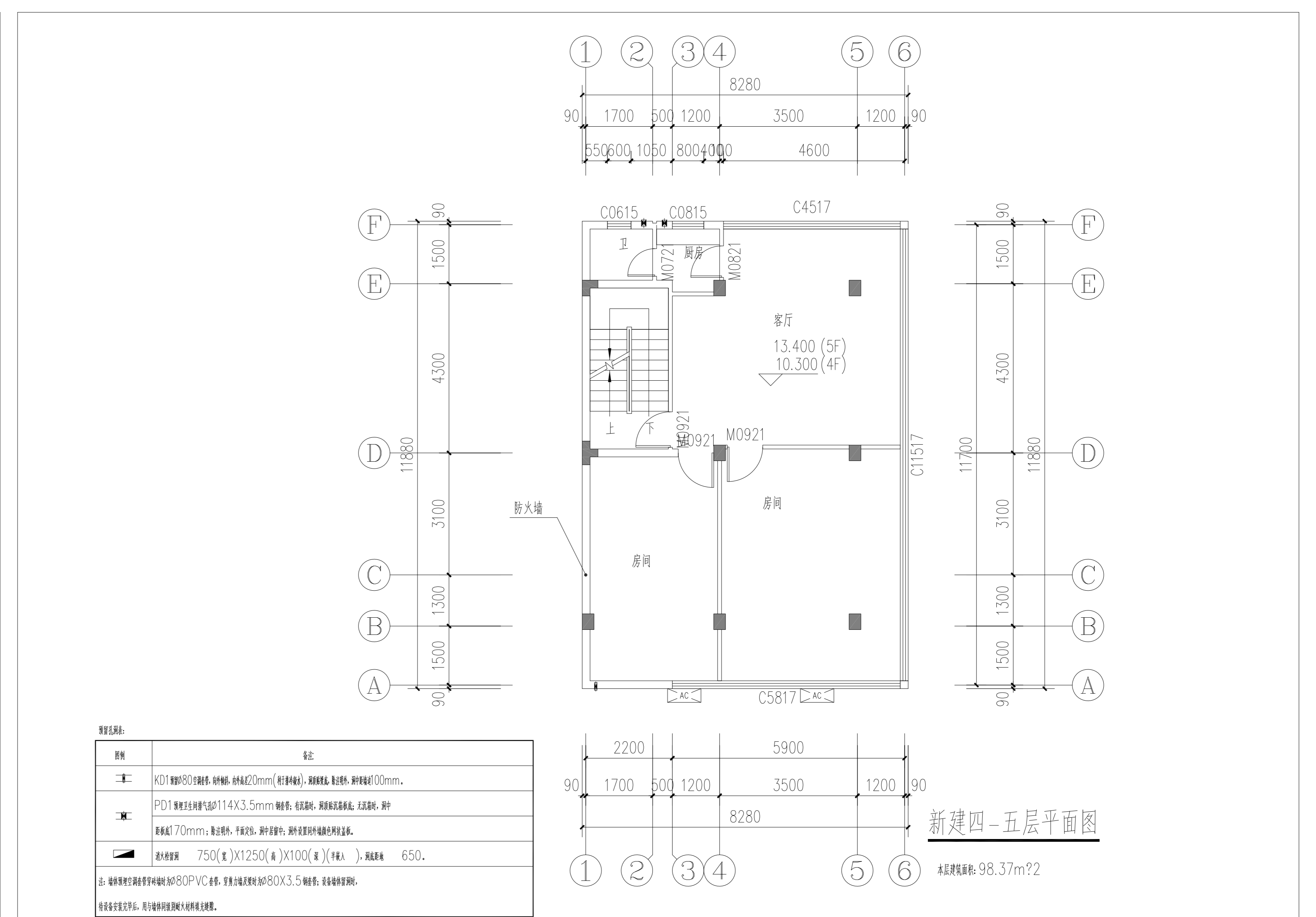
新建四、五层平面图
