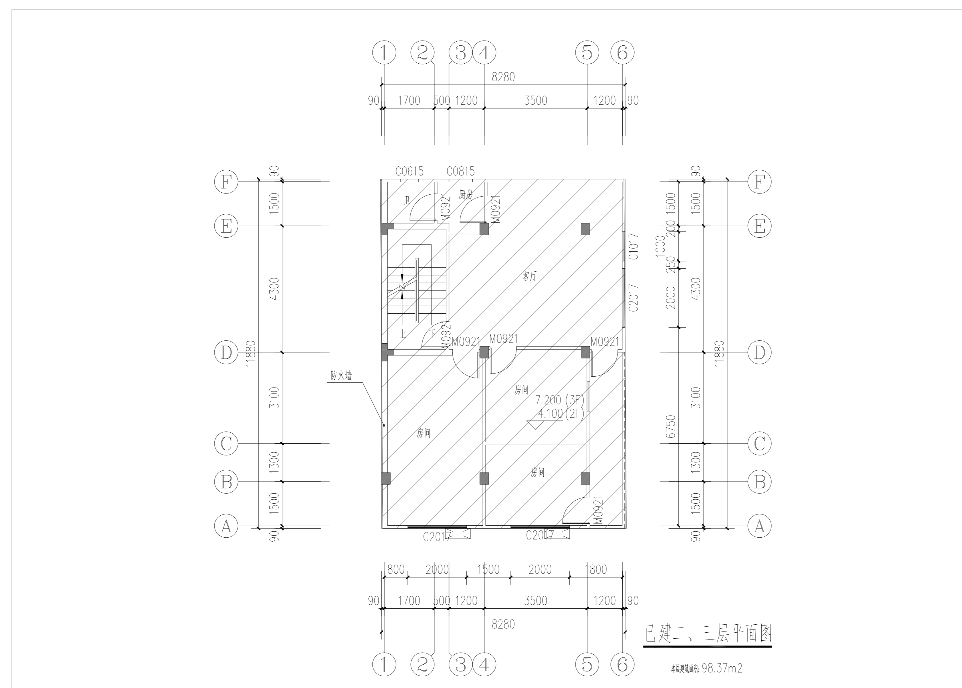
已建二、三层平面图
