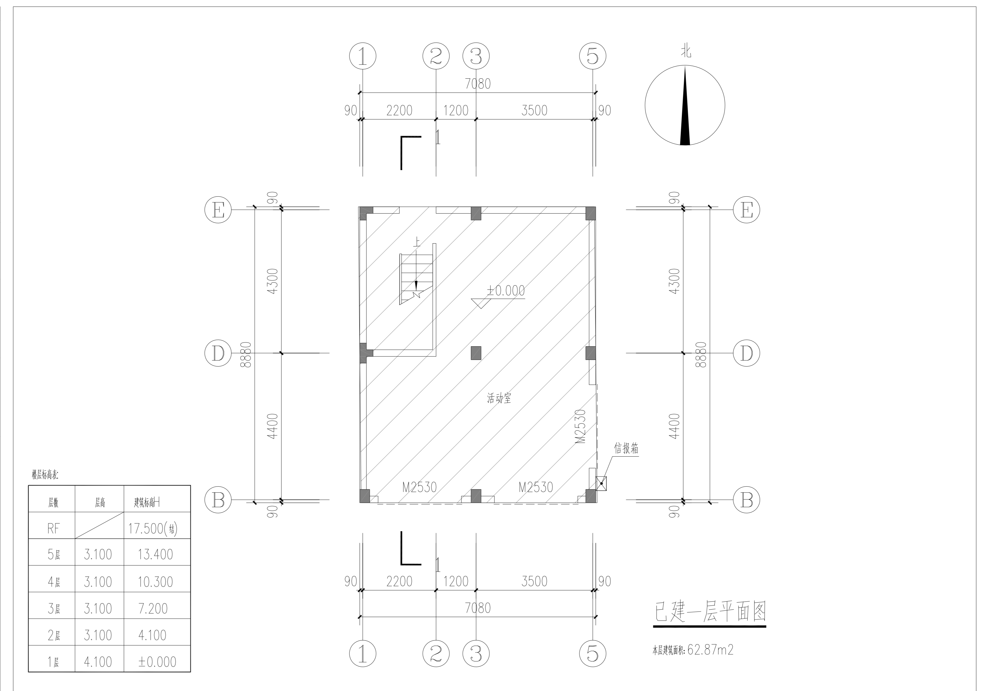
已建一层平面图
