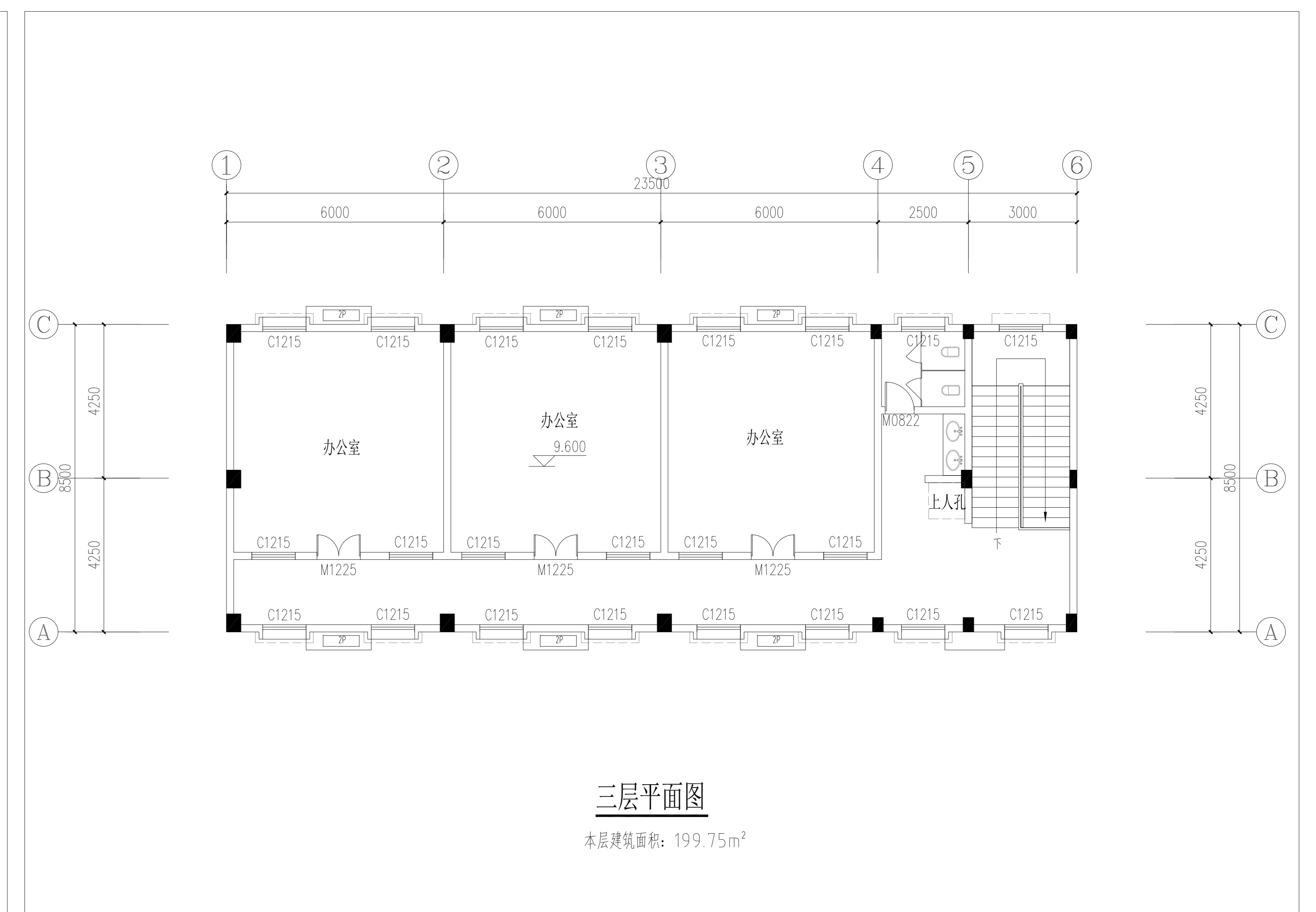
三层平面图
