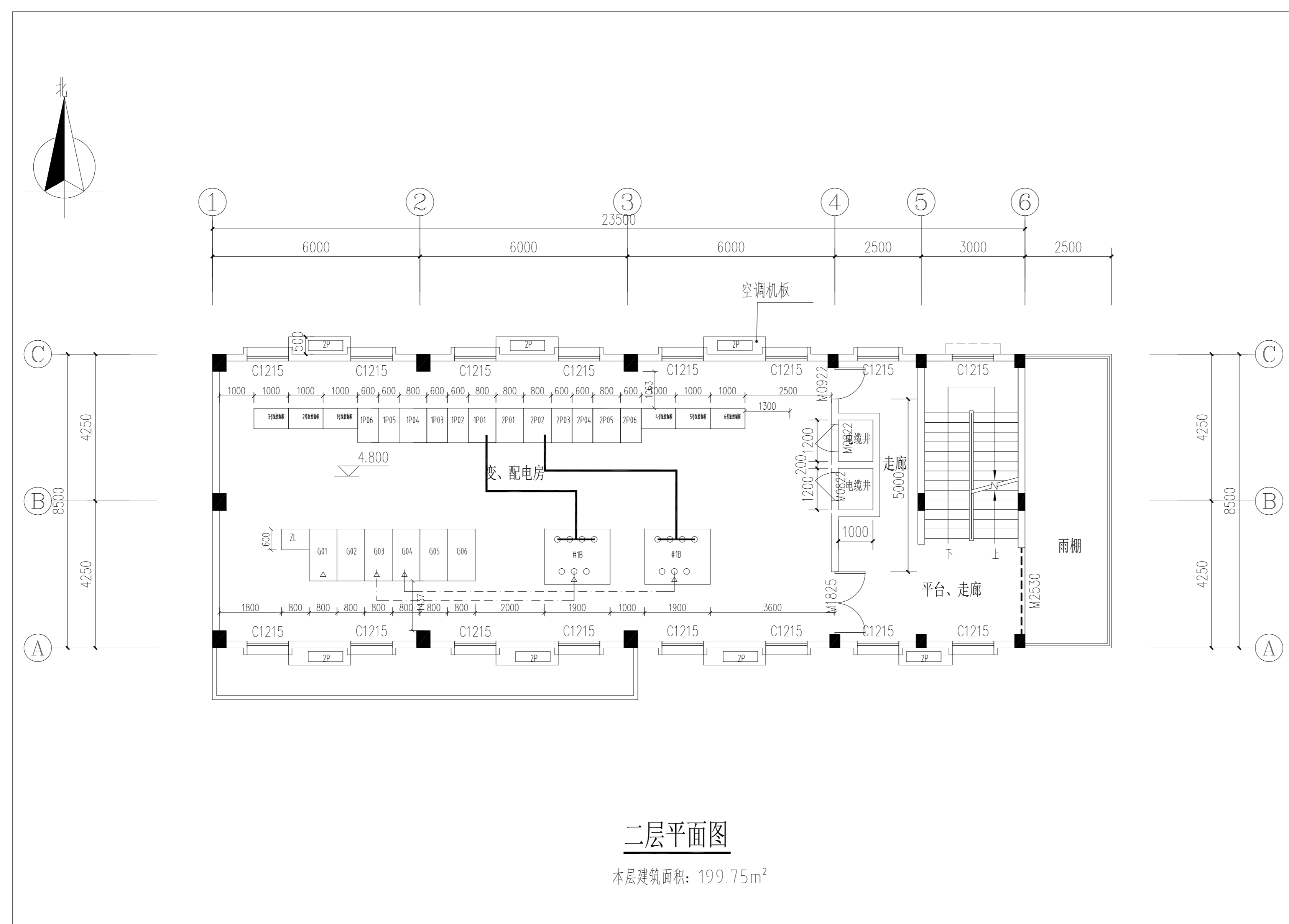
二层平面图
