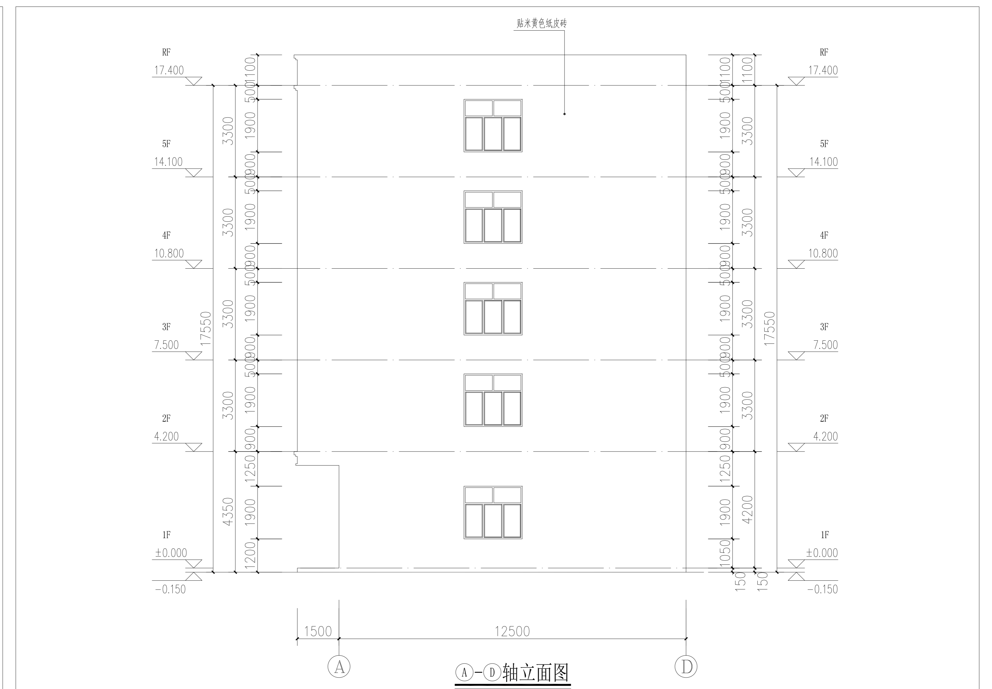
立面图
