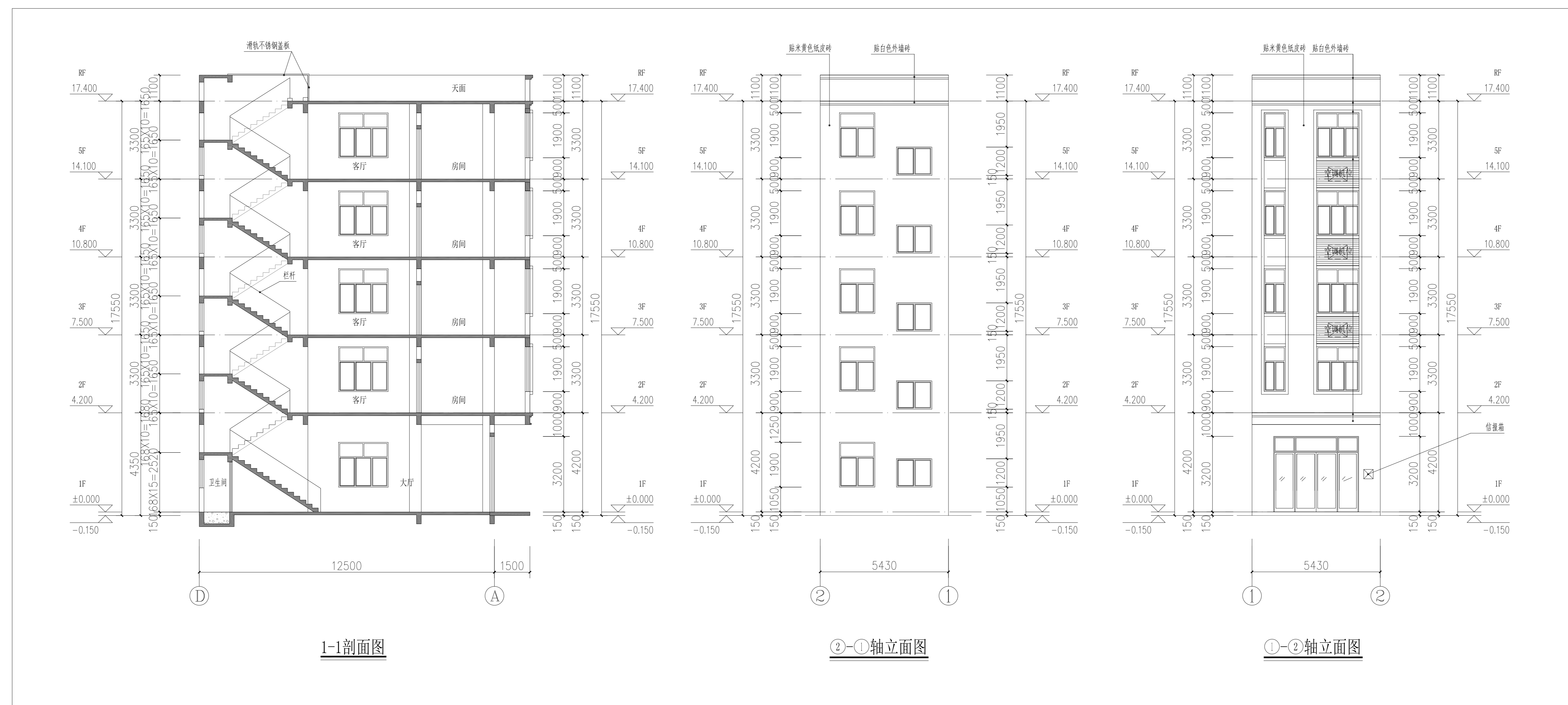
立面和剖面图
