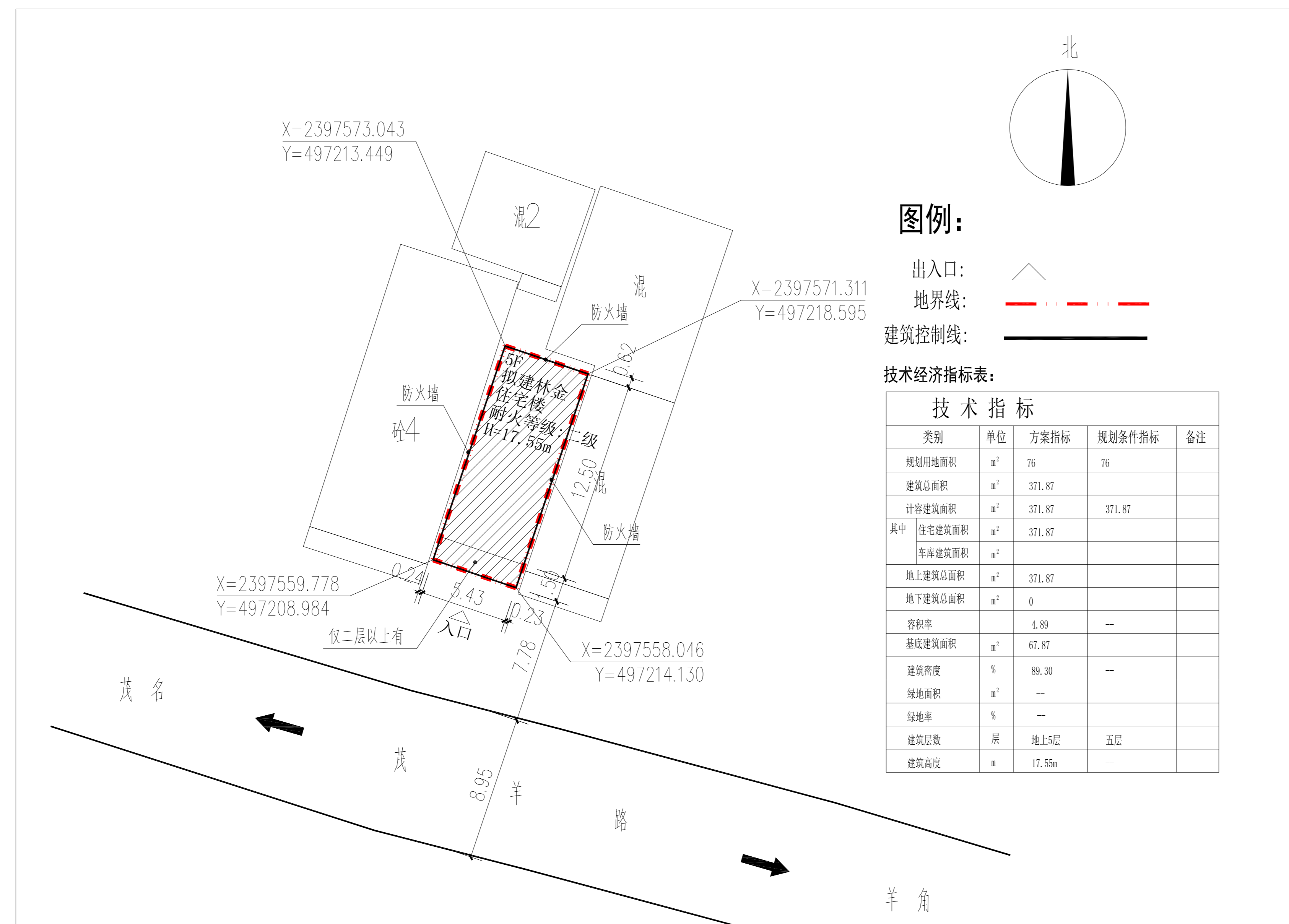
总平面图
