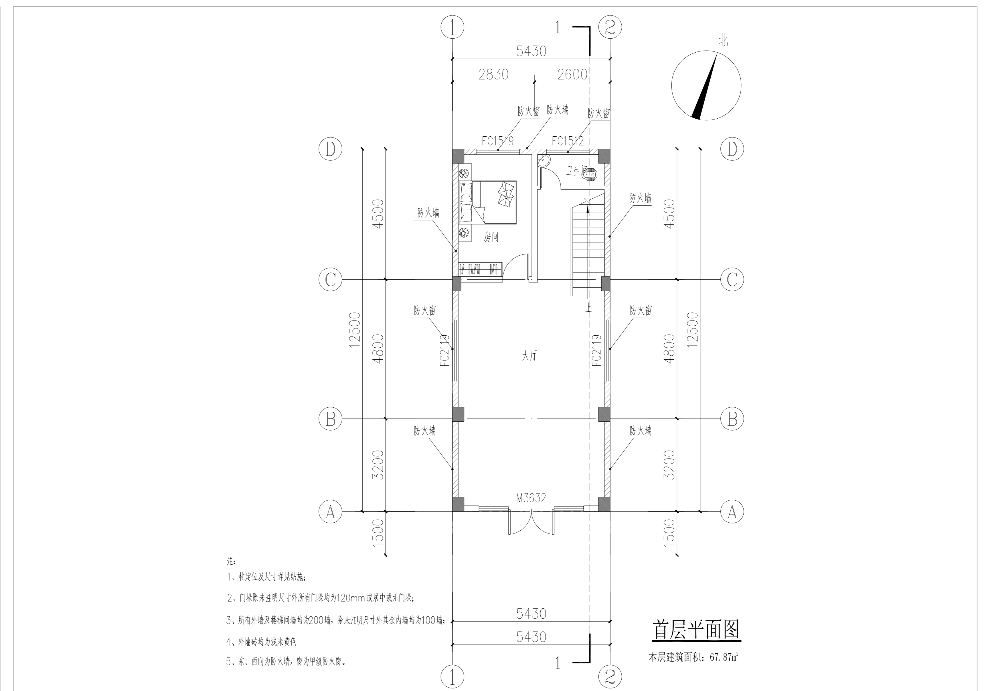
首层平面图
