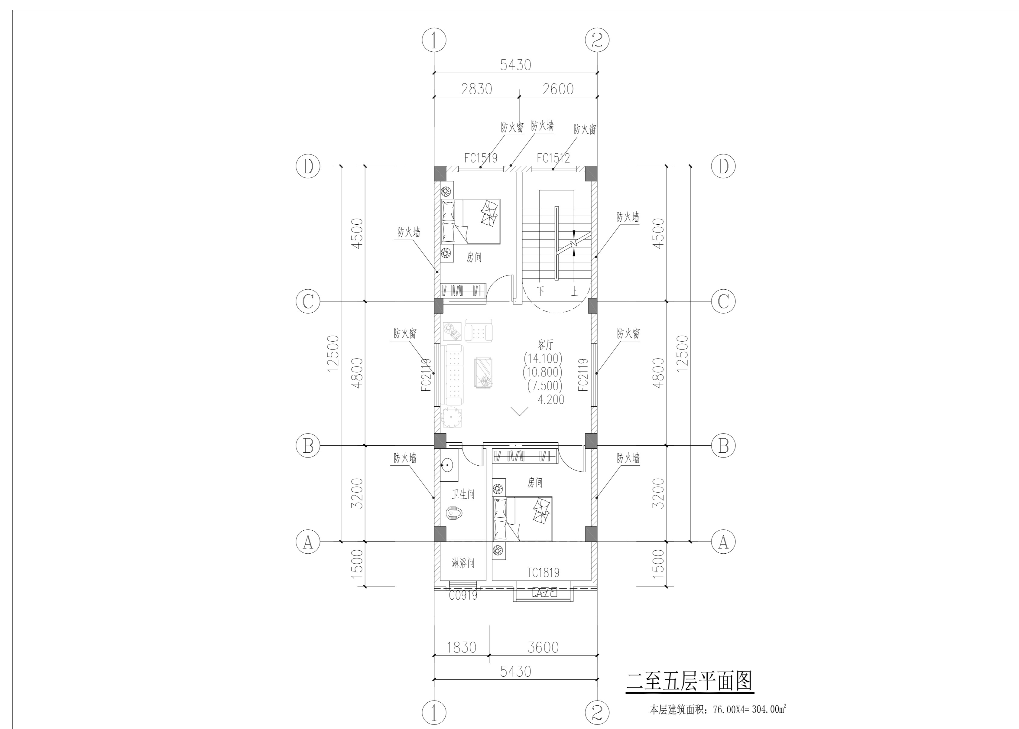
二至五层平面图
