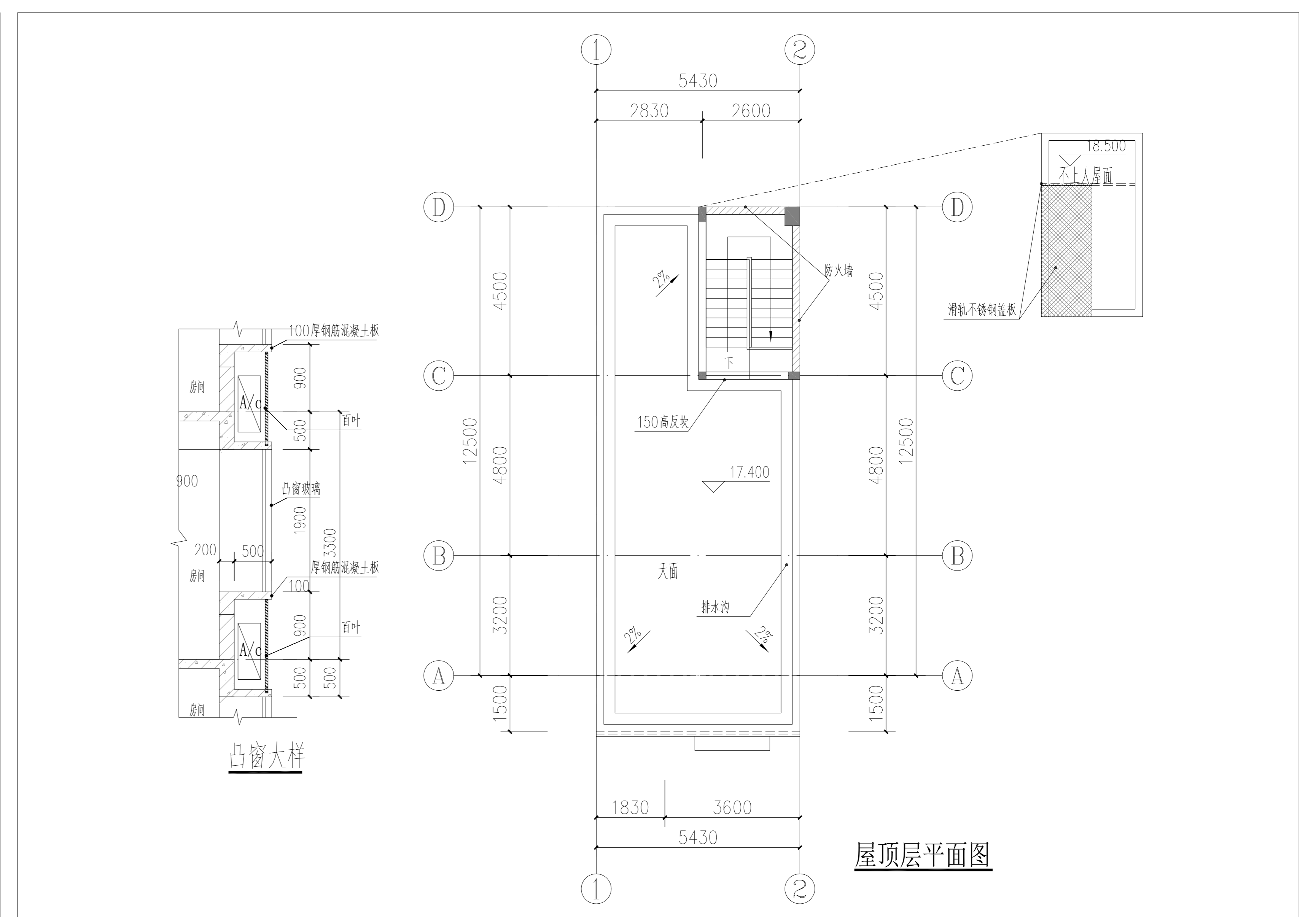
屋顶层平面图
